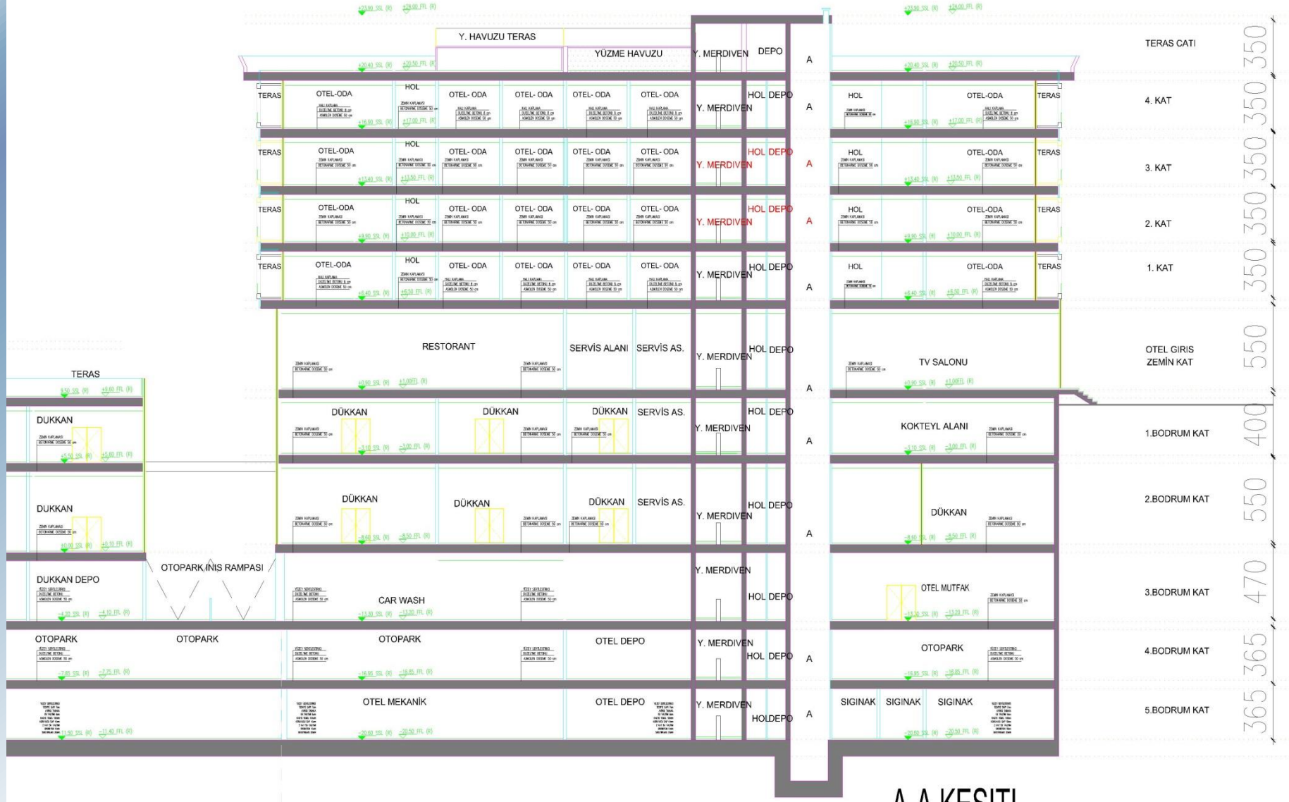
A-A KESİTİ
